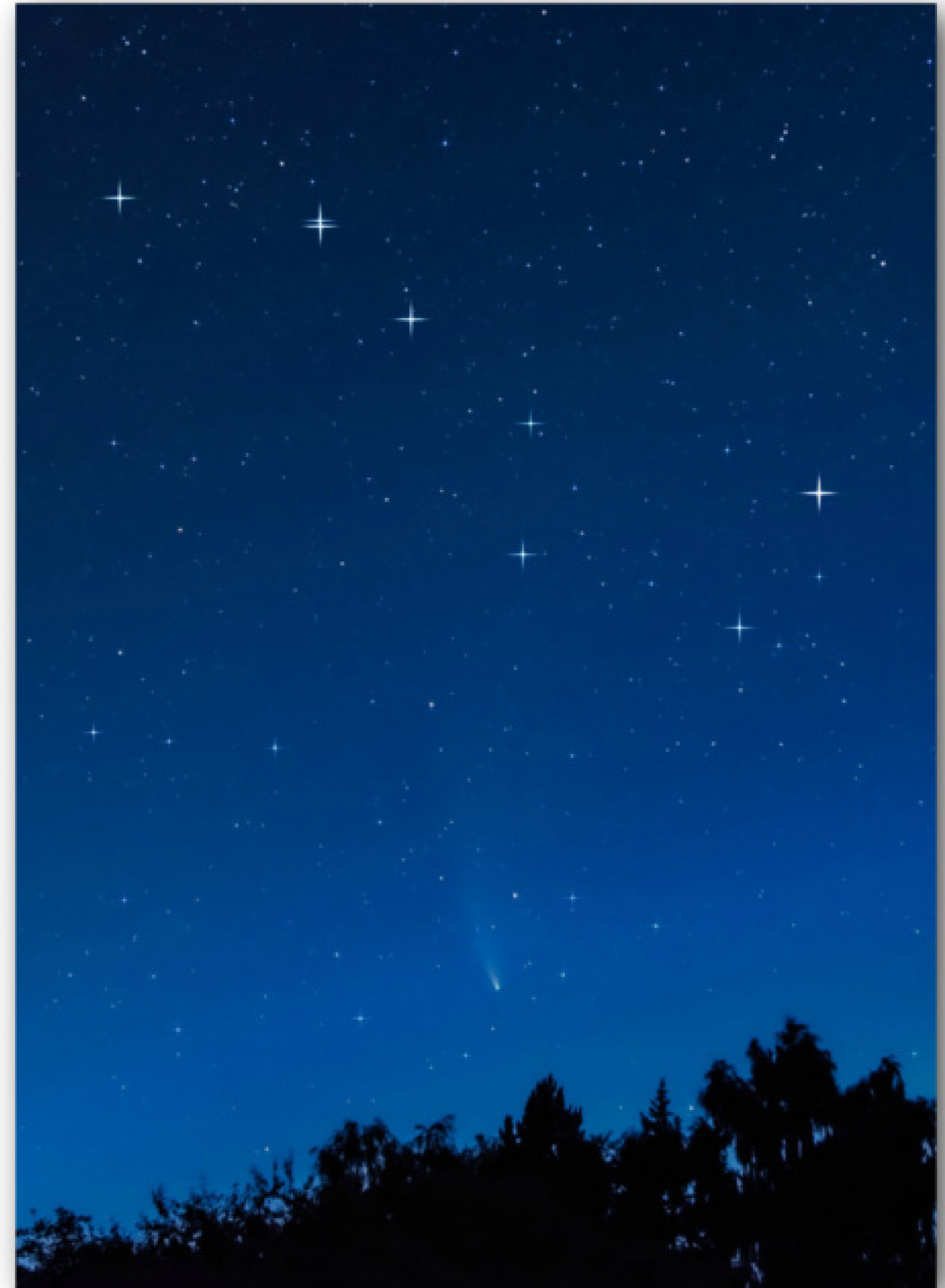
Andromeda Galaxie / M31 mit der elliptischen Galaxie M110 + Komet C/2020 F3 (Neowise) mit dem Sternbild Großer Wagen
