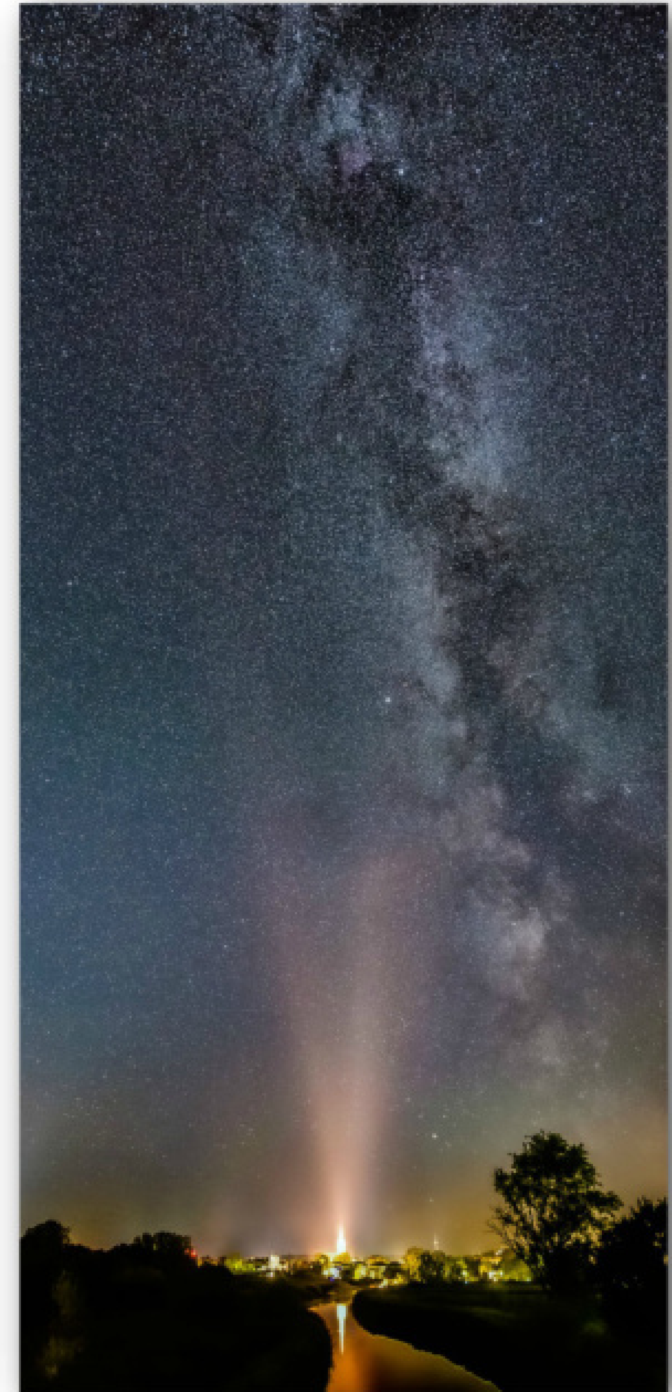
Milchstraße vom Wilseder Berg über der Lüneburger Heide + Milchstraße bei Vollmond über dem Büsenbachtal + Milchstraße über Buxtehude und der Este mit angestrahlem Kirchturm der St. Petri Kirche
